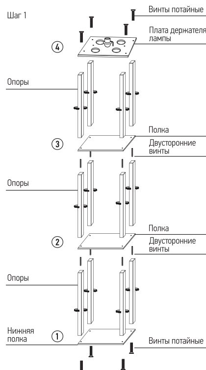
Рис. 1 Сборка светильника ТНО 06КВ-E27
