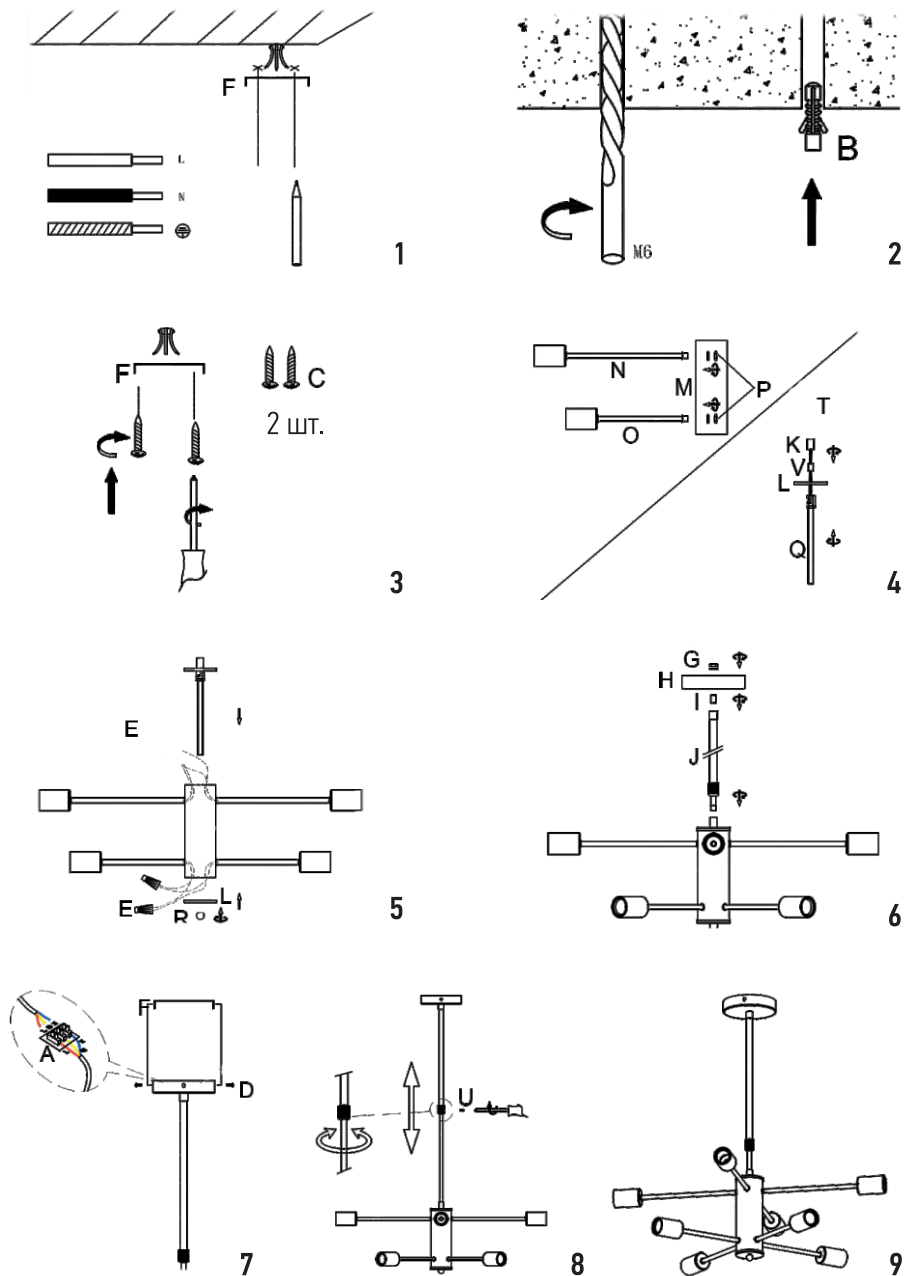
- Рис. 2. Схема подключения LOFT SPUTNIK-8E27-BL, LOFT SPUTNIK-8E27-BLT
